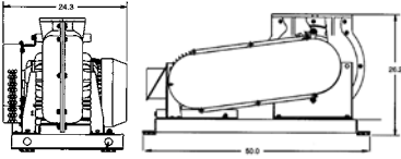
TurboPak C
