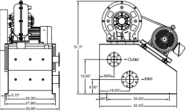
TurboPak C
